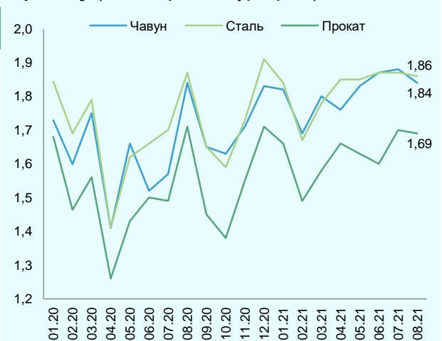
Рис.2.5 Виробництво чавуну, сталі та прокату (дані Укрметалургпром), млн.т
